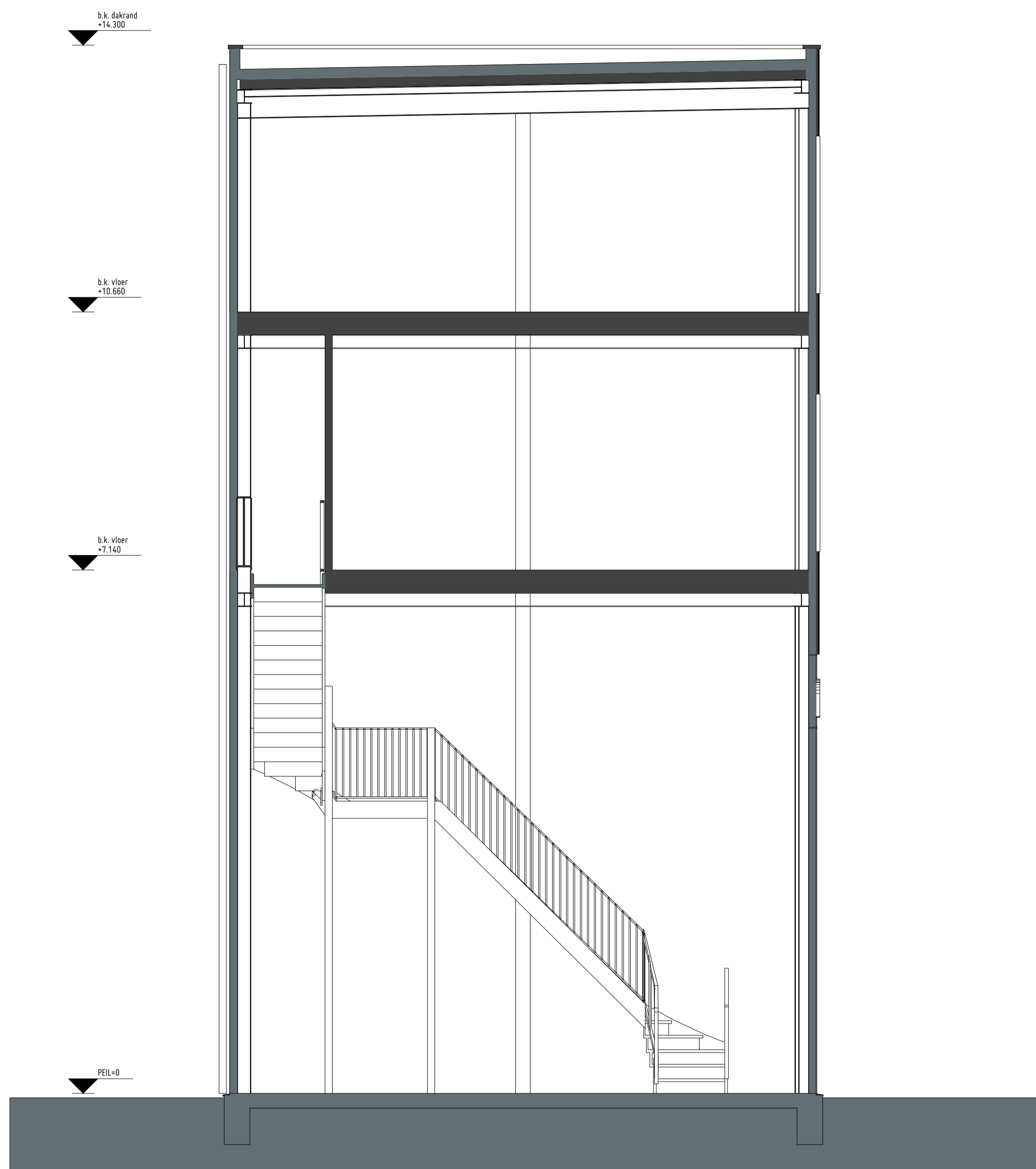
Langsdoorsnede 1:50
