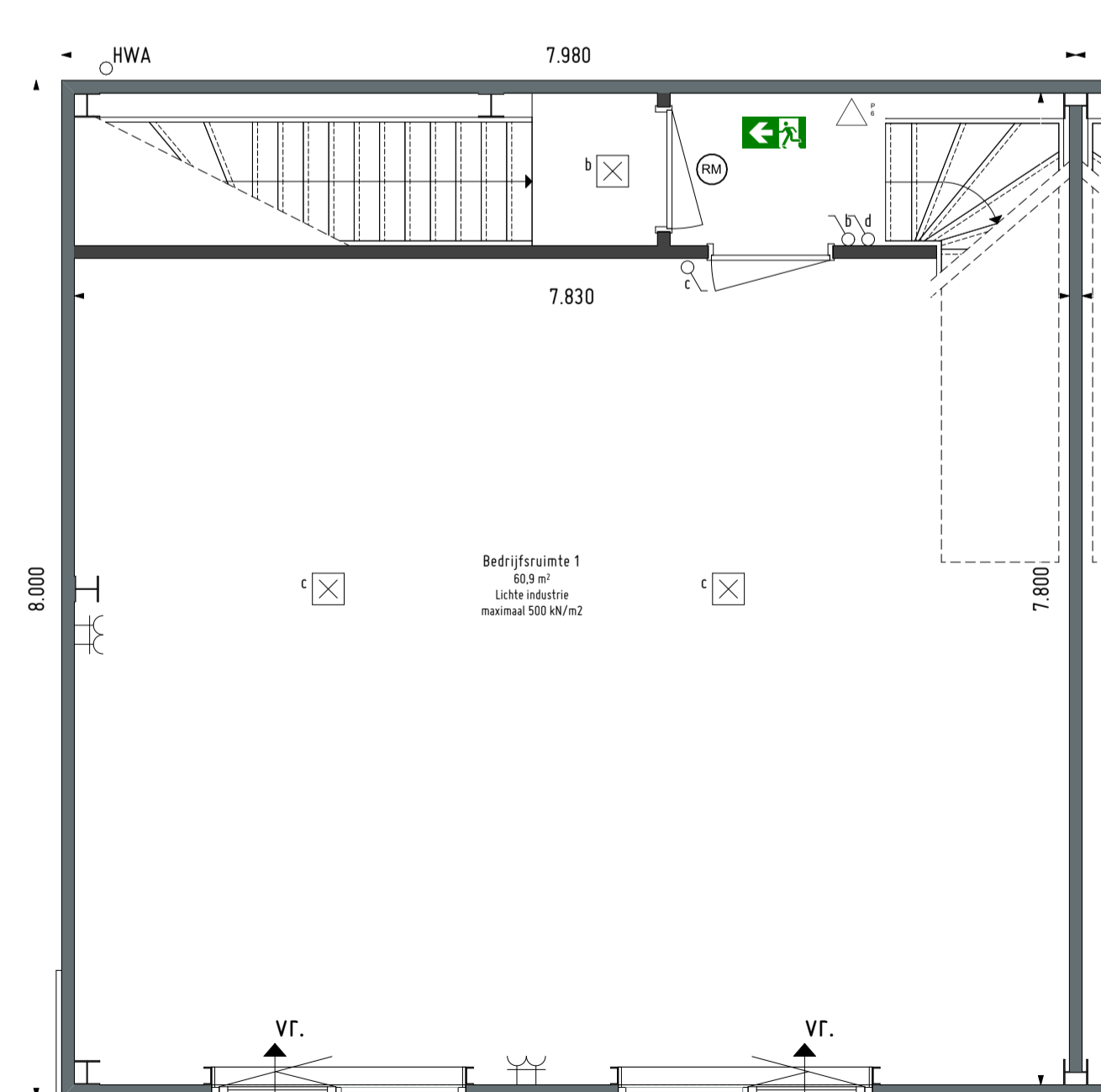
Eerste verdieping, BV0 63,8 m2 1:50
