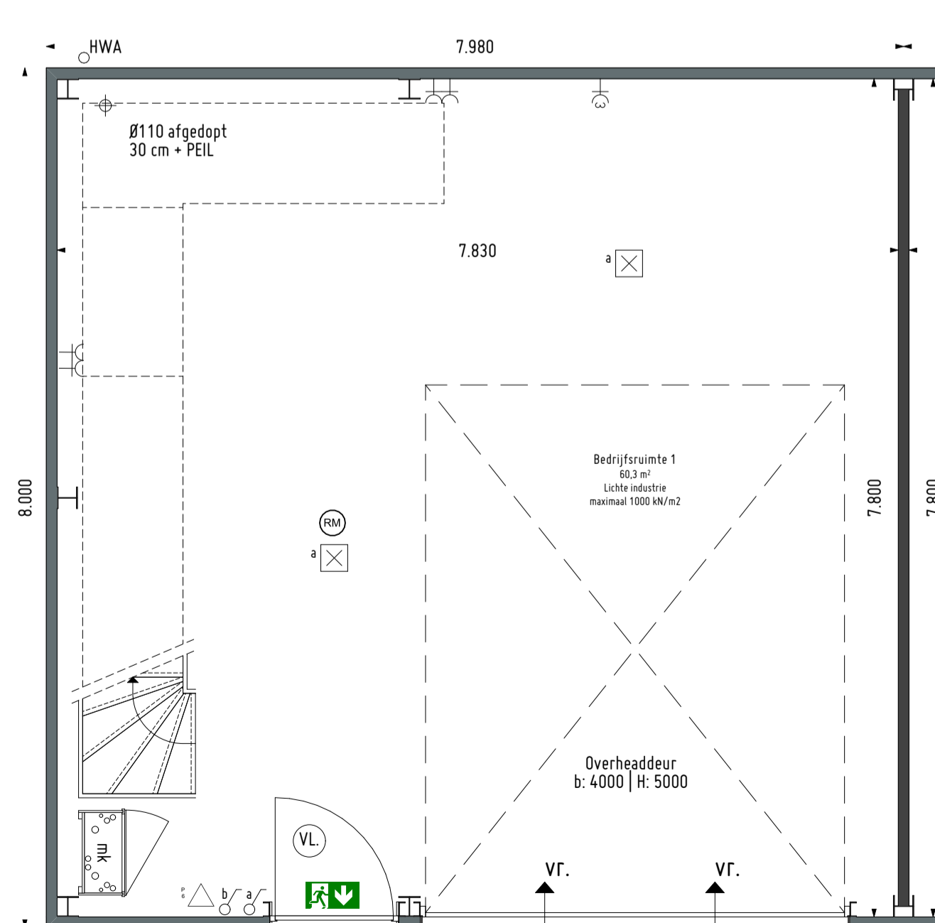
Begane grond, BV0 63,8 m2 1:50
