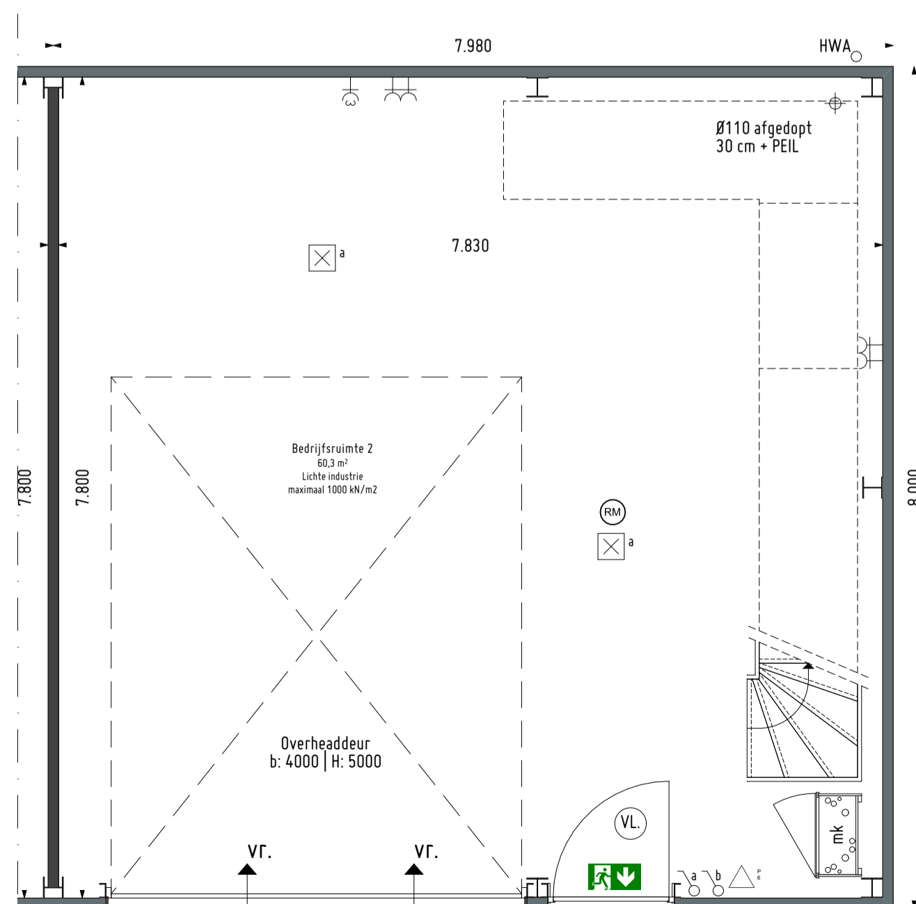
Begane grond, BVO 63,8 m2 1:50
