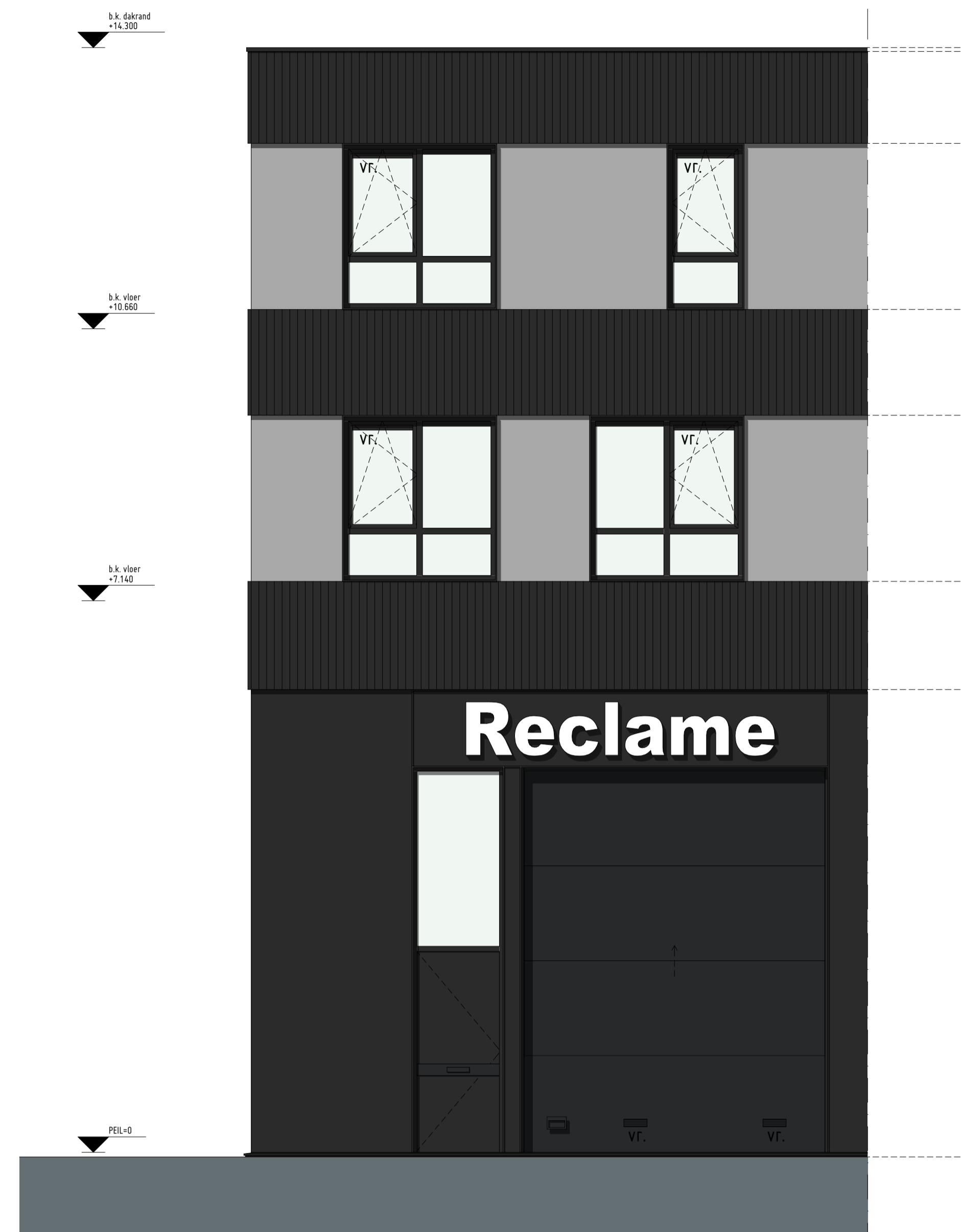
Voorgevel 1:50
