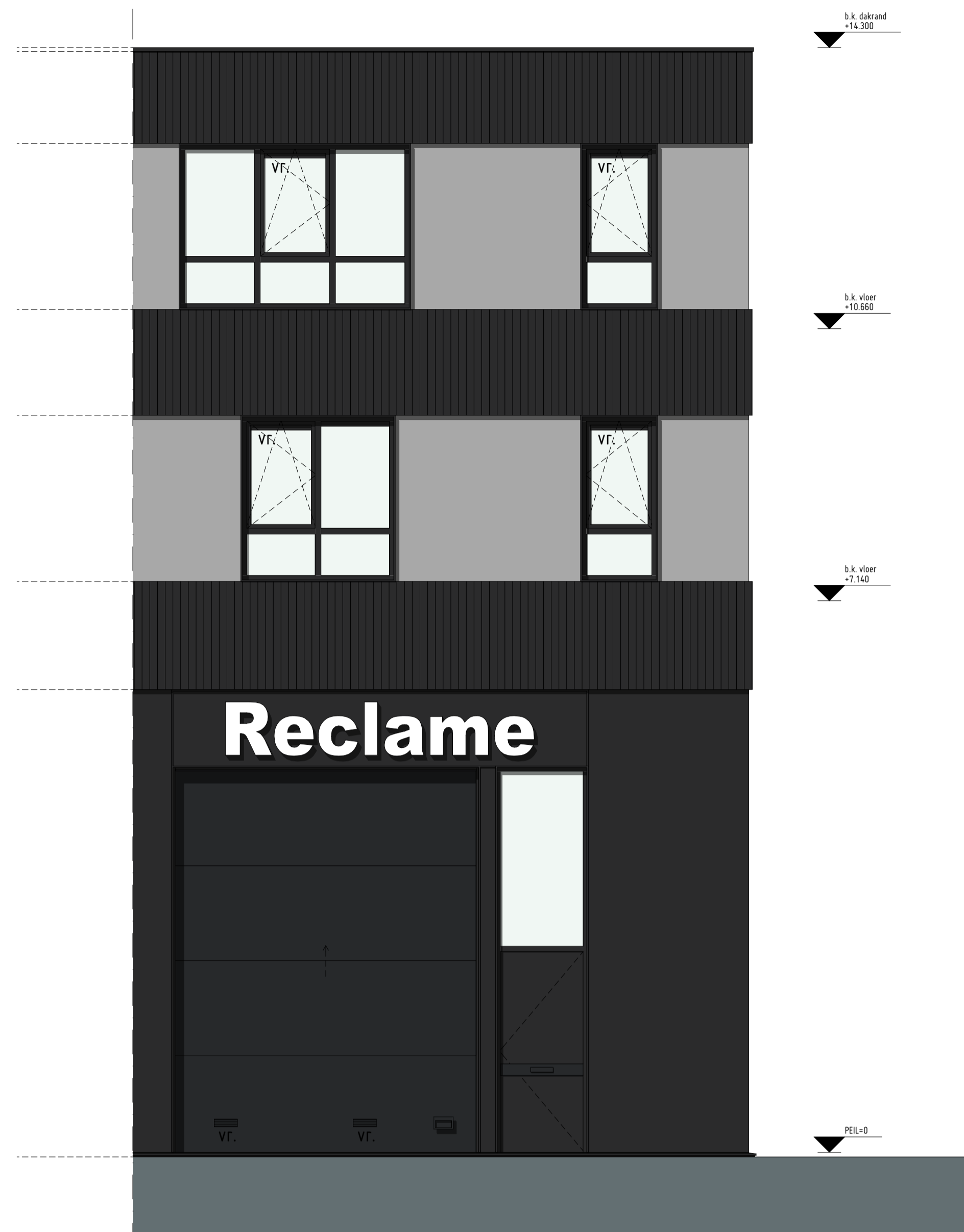
Voorgevel 1:50
