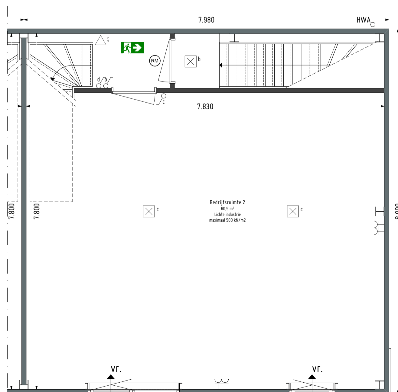
Eerste verdieping, BVO 63,8 m2 1:50
