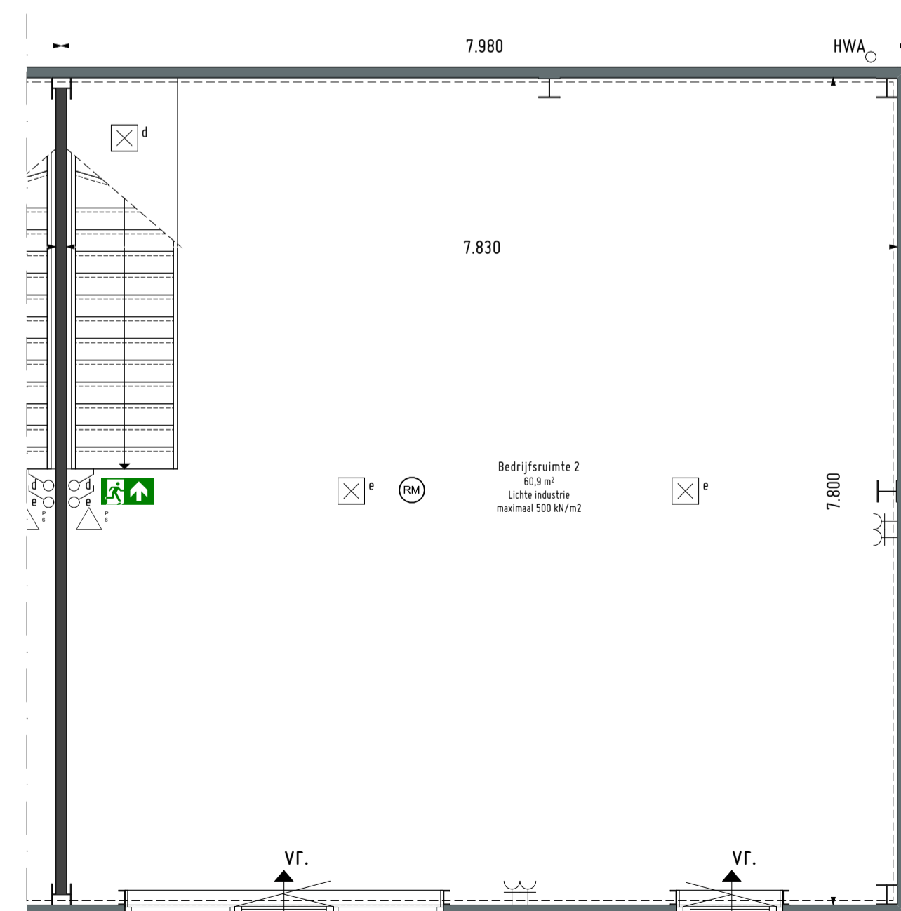
Tweede verdieping, BVO 63,8 m2 1:50
