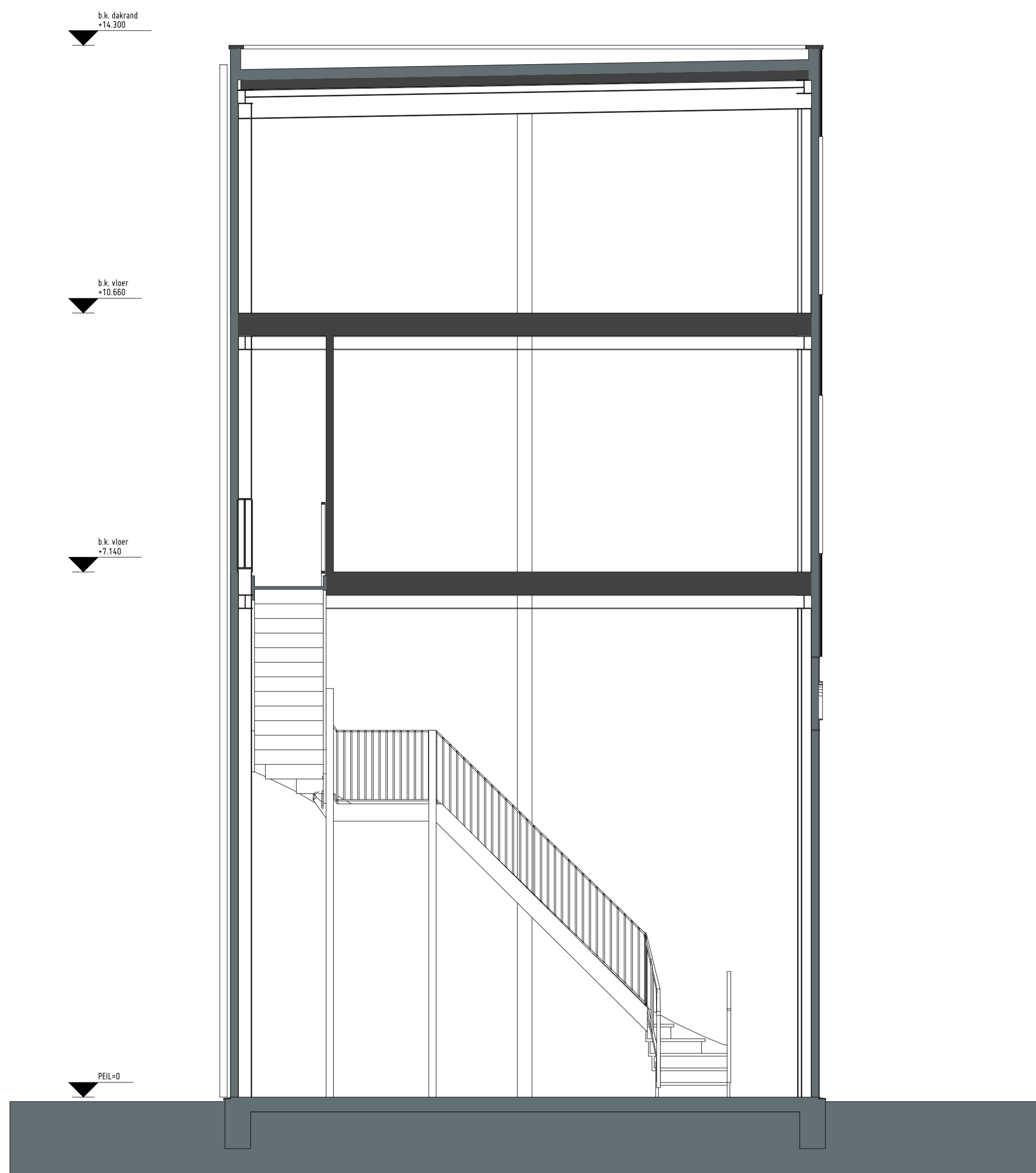
Langsdoorsnede 1:50
